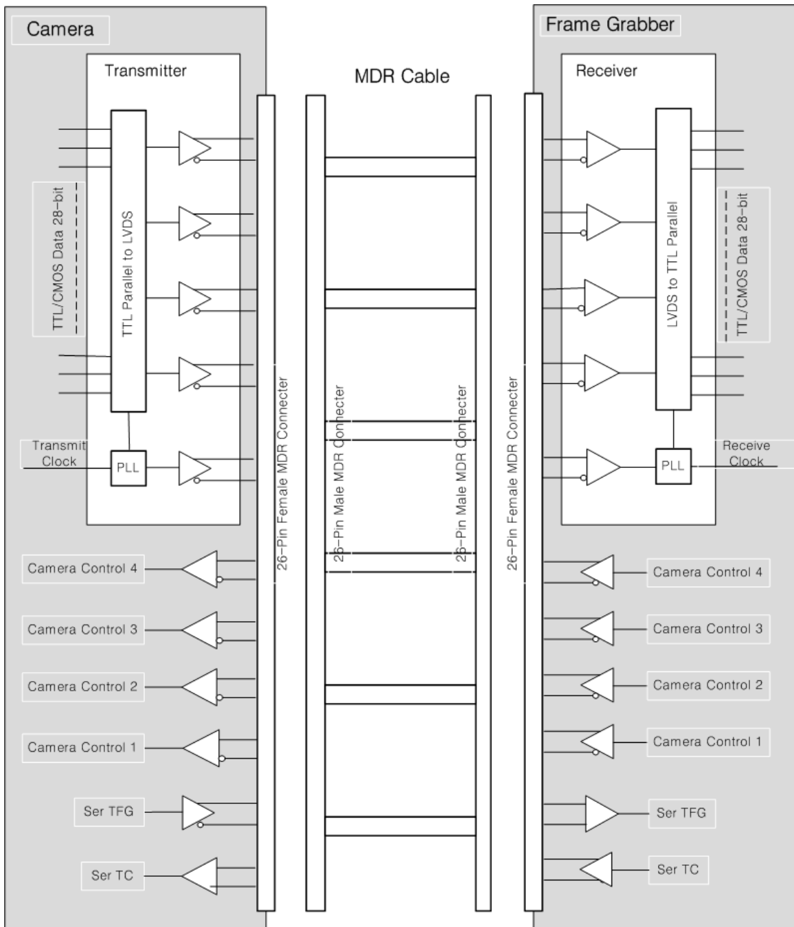
[그림 2-2. Base Camera Link 블록도]
