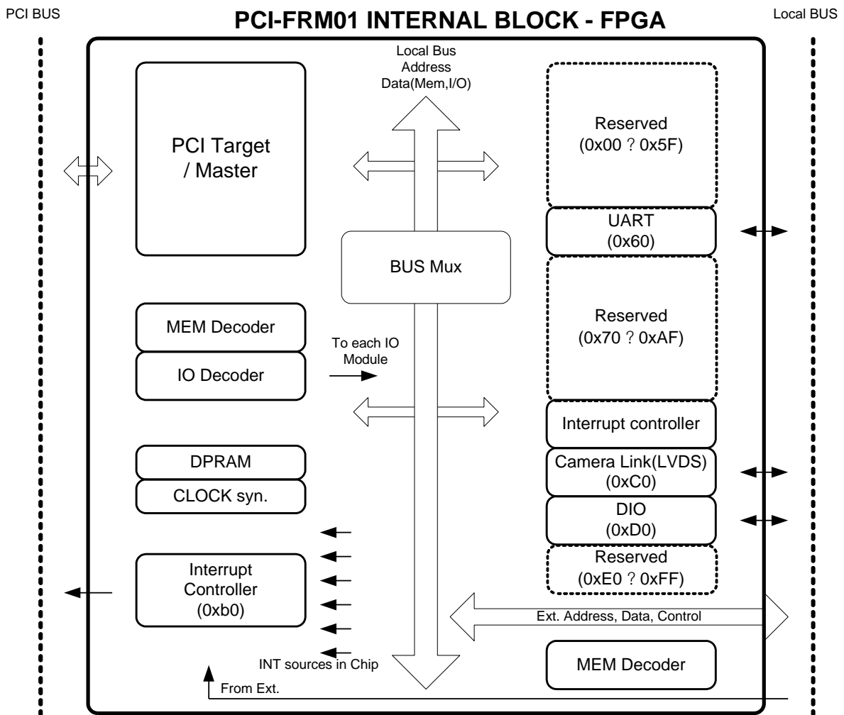
[그림 2-1. PCI-FRM01 기능 블록도]
