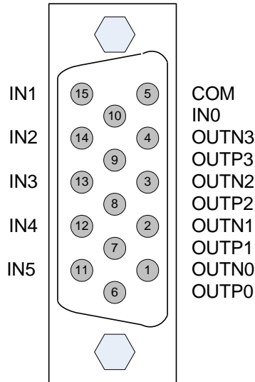
[그림 3-5. P1 DSUB 15PIN Pin-out]
