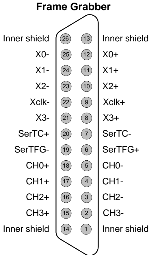
[그림 3-3. PCI-FRM01 J1 Connector Pin-out]
