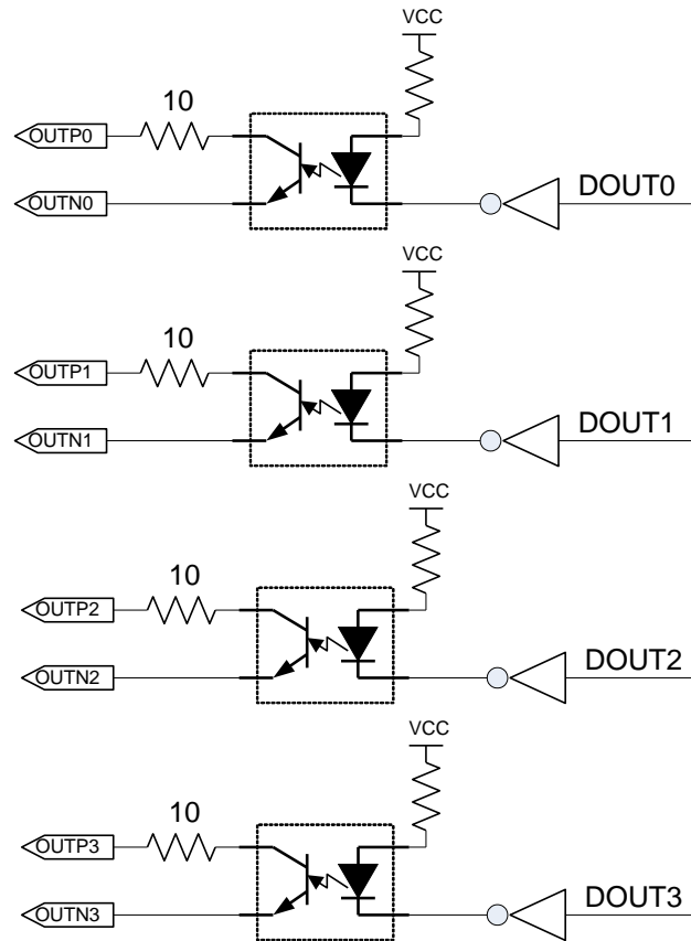
[그림 3-7. 포토 커플러 디지털 출력 회로]
