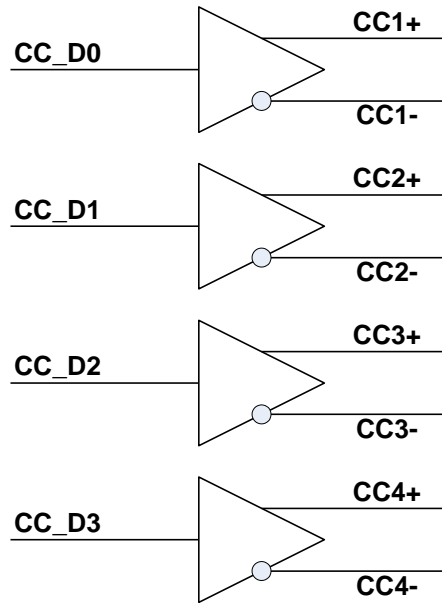
[그림 2-6. Camera Control LVDS Digital 출력 회로]
