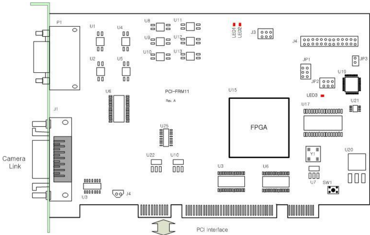
[그림 3-1. PCI-FRM01 외형도]
