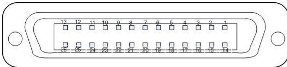
[그림 2-5. MDR-26 Connector (Female) Pin Map]
