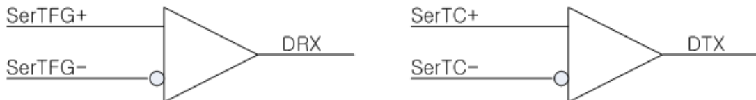
[그림 2-7. Serial Communication LVDS Digital 출력 회로]
