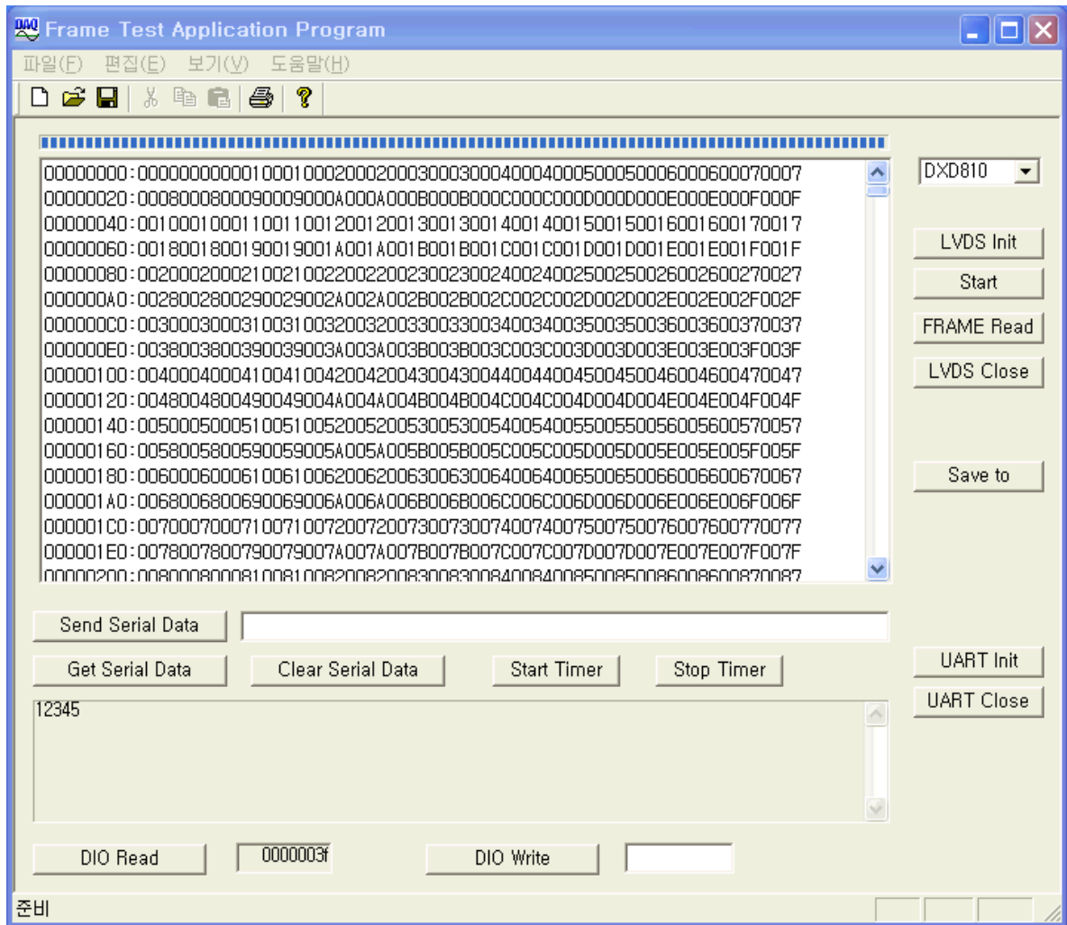
[그림 5-1. 샘플 프로그램 “FrmTest.exe” 실행화면]
