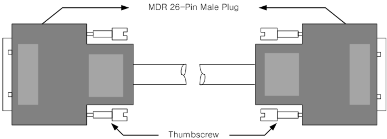
[그림 2-3. MDR-26 Camera Link Straight Cable]
