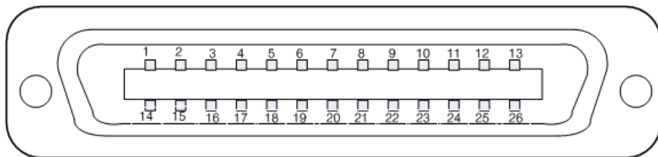
[그림 2-4. MDR-26 Cable (Male) Pin Map]
