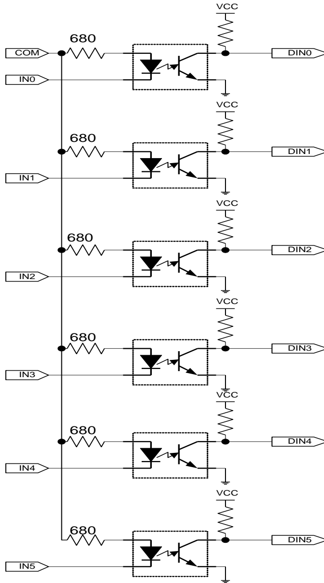
[그림 3-6. 포토 커플러 디지털 입력 회로]
